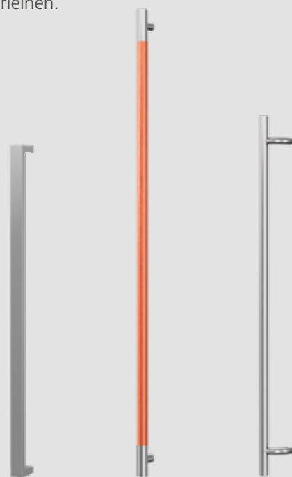
Außengriff G120gf-E, Länge 1.050 mm
