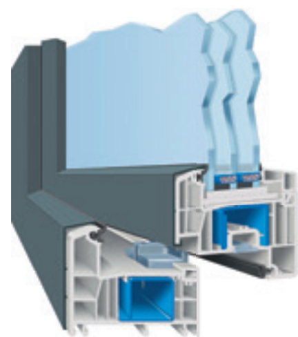
AFINO-top AD (Sistema de doble junta)
