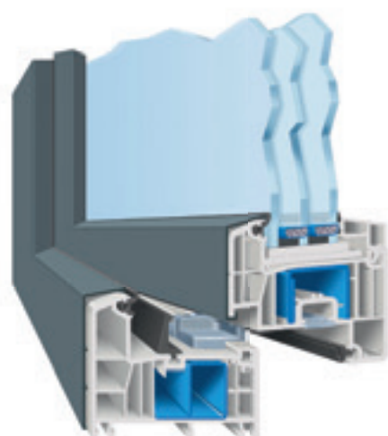
AFINO-top MD (Sistema de tres juntas)
